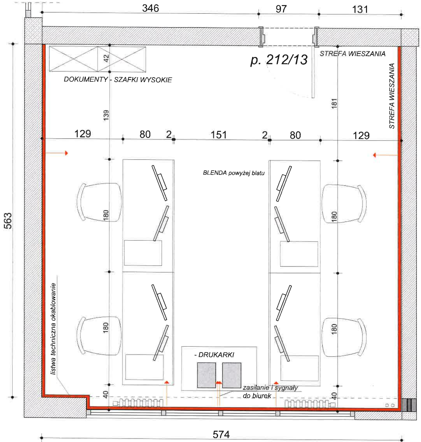
pokój pracowniczy - RZUT
